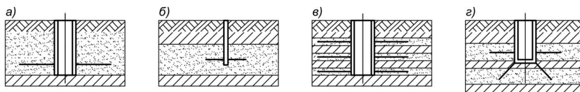
Зураг 2. Цацраган ус татамжийн огтлол
