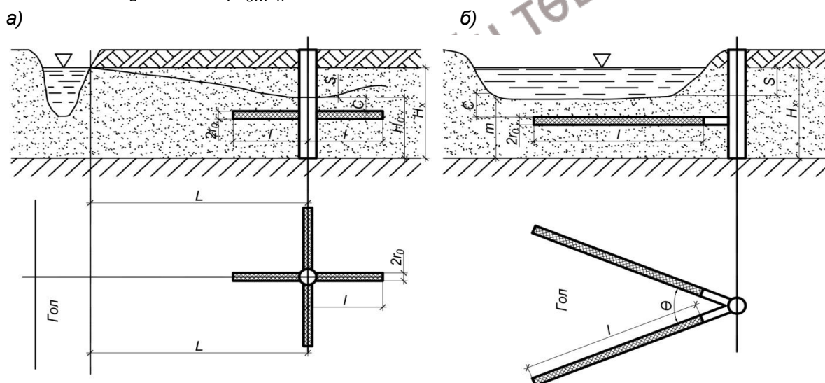
Зураг 3. Цацрагт ус татамжийн тооцооны схем
